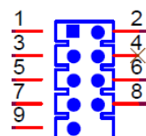
BMC_CN1
