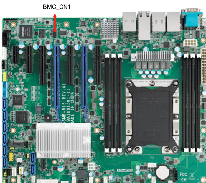
BMC_CN1
