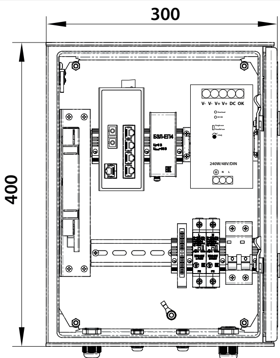
Устройство шкафа (дверь открыта на 90°)
