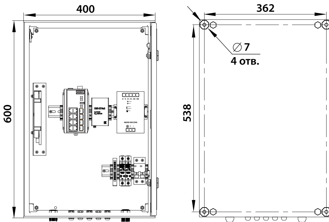
Устройство шкафа (дверь открыта на 90°)
