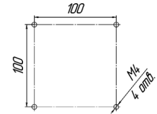
Рисунок 3 – Установочные размеры для крепления на стену
