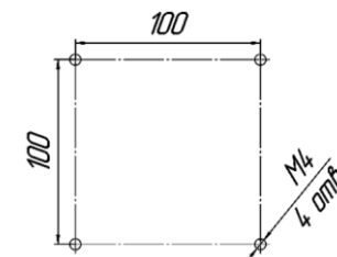
Рисунок 3 – Установочные размеры для крепления на стену
