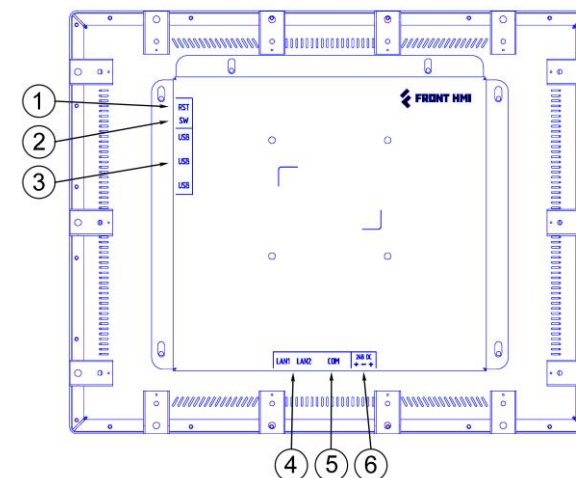
Рисунок 4 – Внешний вид тыльной стороны устройства
