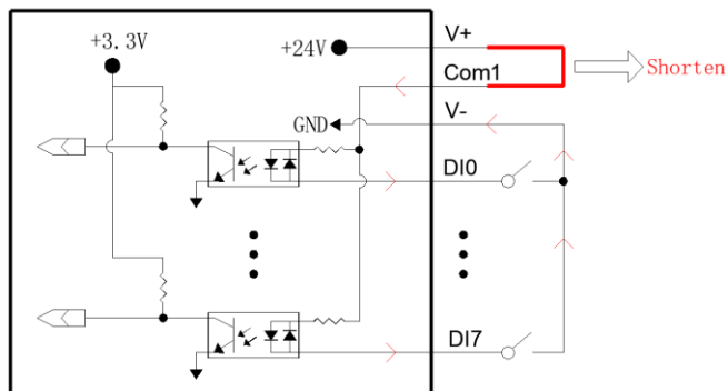
Figure 22 DI NPN wiring solution
