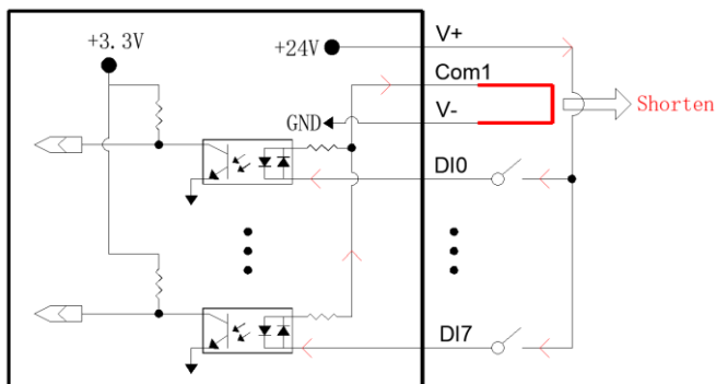
Figure 23 DI PNP wiring solution
