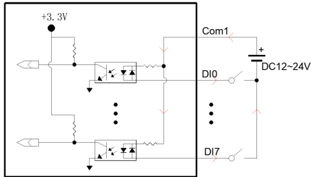
Figure 8 DI NPN wiring solution
